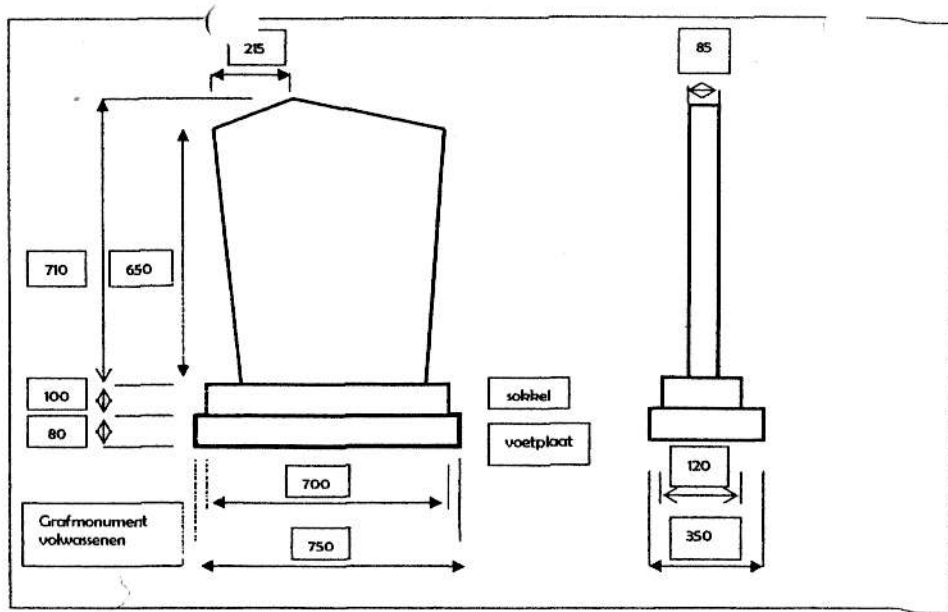
Grafmonument volwassenen
