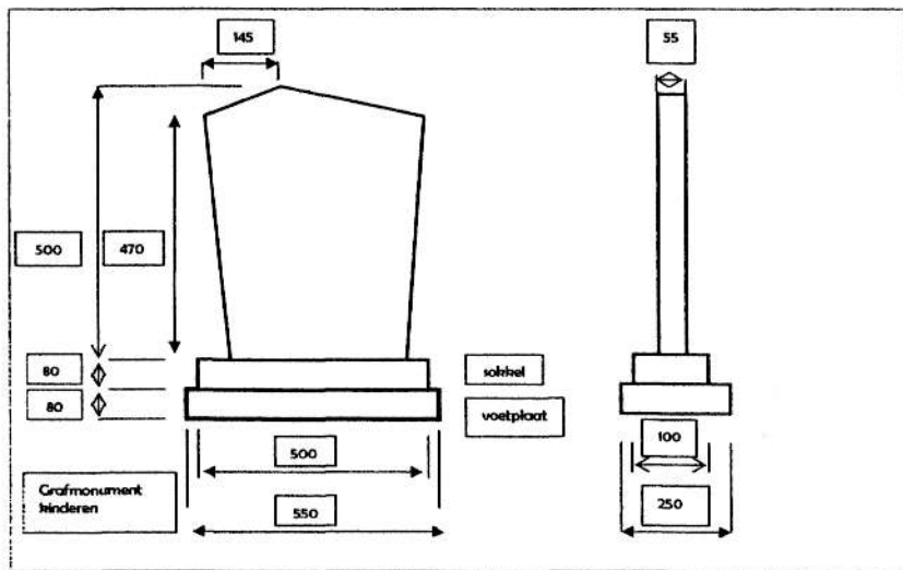
Grafmonument kinderen
